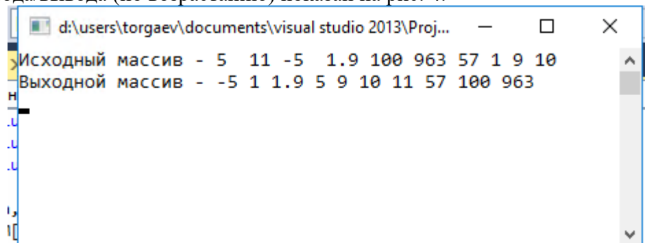
Рис. 4. Пример выполнения программы
